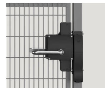
SCHMERSAL AZM201 Fästen som passar många typer av AZM på många slags portar och dörrar.
