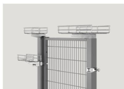
KABELSTEGE Det är lätt att fästa konsoler på stolparna eller Smart Fix-fästet, för kabelstege med en bredd på 100 mm eller 200 mm.
