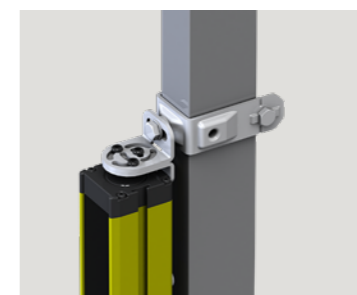
FÄSTE FÖR LJUSBOM Montera olika typer av ljusbommar direkt på stolpen med Smart Fix-fästet.
