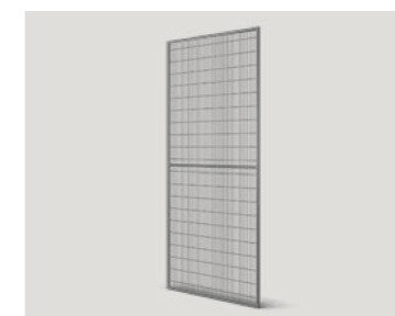
PANEEL ST20 Een sterk gaaspaneel met een maaswijdte van 100x20 mm en een draaddikte van 3 mm, bevestigd op een frame van 19x19 mm.
