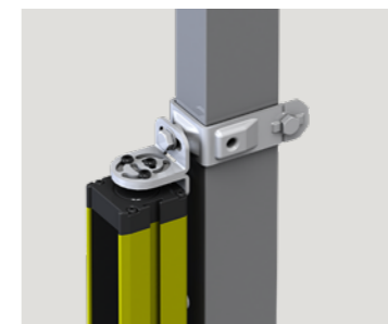
BEUGEL VOOR LICHTSCHERM Plaats verschillende soorten lichtschermen rechtstreeks op de Troax-staanders met de verstelbare Smart Fix beugel.
