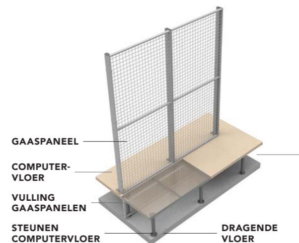
Een voorbeeld van een gaasvulling tussen de vaste vloer en de computervloer.
