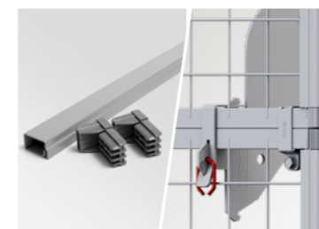
11 CUT-PROFIEL VOOR AANPASSINGEN IN HOOGTE Dit is een makkelijke en flexibele oplossing om tijdens de installatie de hoogte van gaaspanelen aan te passen en de sterkte van het systeem te behouden.
