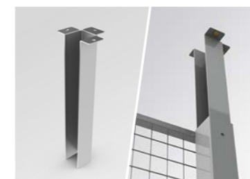
10 PLAFONDSTEUN 80x80 Wordt gebruikt om een hoge wand aan het plafond te bevestigen. Voorzien van een telescopisch ontwerp om in te spelen op constructiebeweging.
