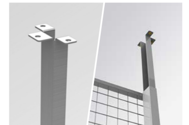
6 PLAFONDSTEUN 60x40 Wordt gebruikt om een hoge wand aan het plafond te bevestigen. Voorzien van een telescopisch ontwerp om in te spelen op constructiebeweging.
